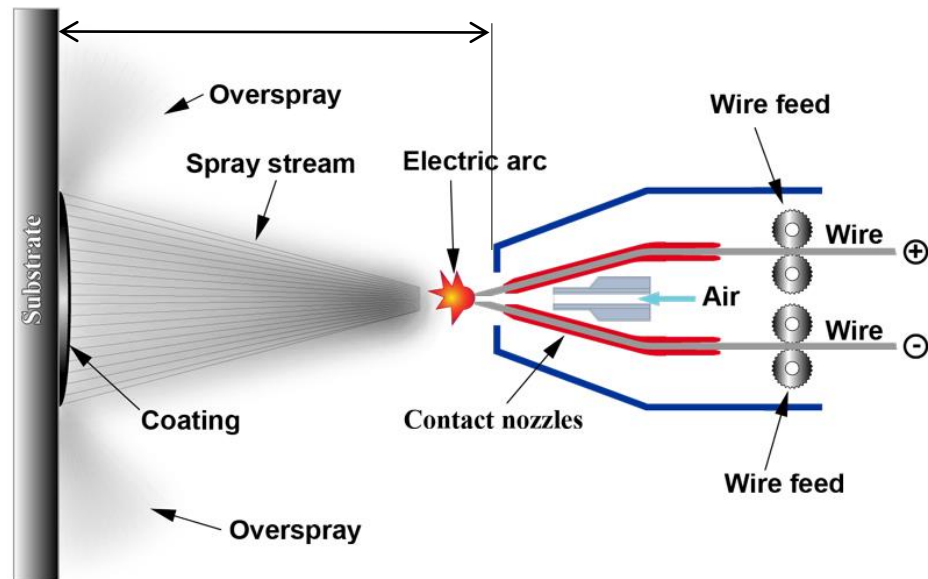
Métallisation au pistolet à arc électrique (AS): Technique
